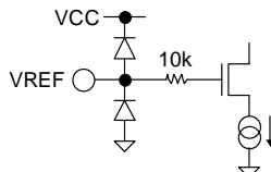
Fig.41 VREF
